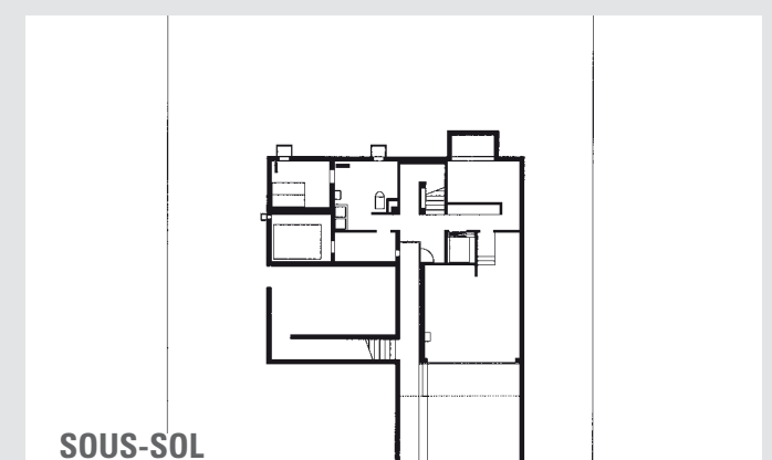
ÉTAGE
